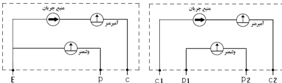
شکل (۲): دستگاه ارت سنج نمونه (سه سیمه)
