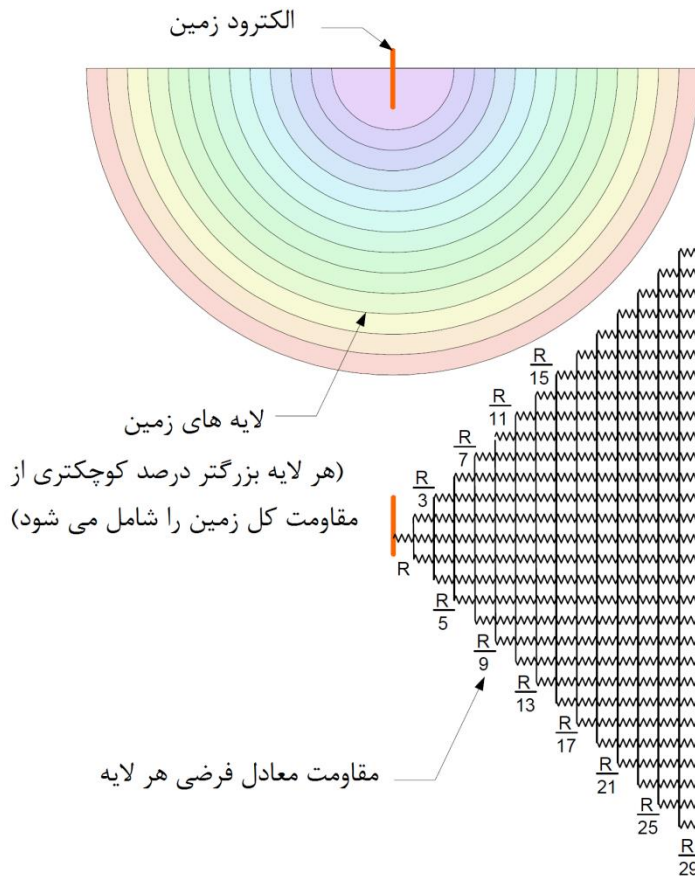
شکل (۱۷): مدار معادل پوسته‌های هم‌پتانسیل طراف یک الکترود
