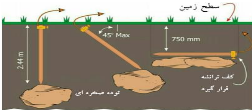
شکل (۶-۲): صورت‌های مجاز اجرای الکتروودهای میله‌ای (NEC : 2014, Art: 250.53)
