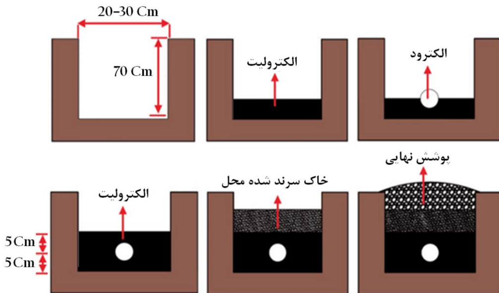
شکل (۷-۲) : نحوه اجرای الکترود افقی با الکترولیت
