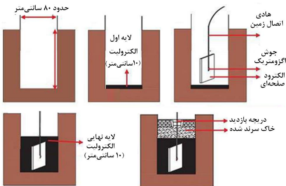
شکل (۹-۲): اجرای الکتروود صفحه‌ای با الکترولیت
